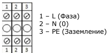
Рис.2. Блок внешних соединений котла.
